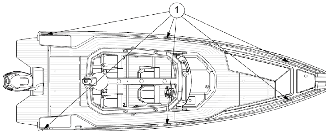
(1) Anschlagpunkte
